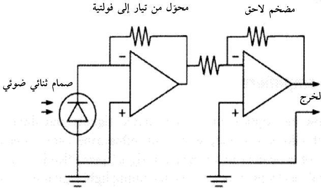
الشكل 5-6 محوّل (ليف بصري) تماثلى
